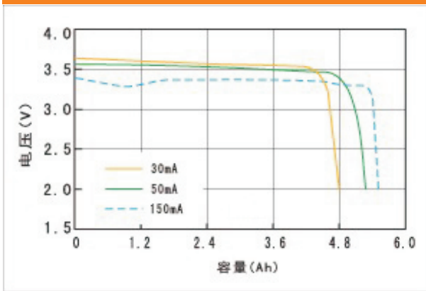
150℃放电曲线
