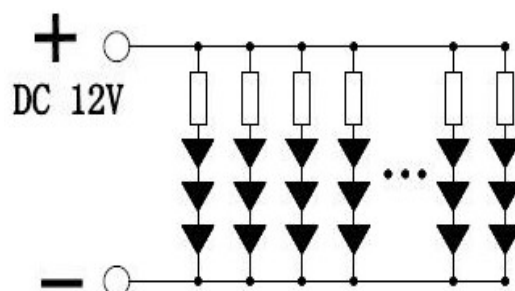
Рис. 2 Принципиальная схема
