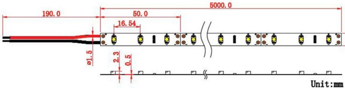
Рис.1 Основные размеры
