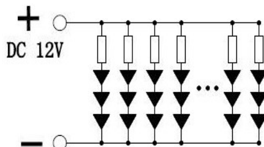
Рис. 2 Принципиальная схема
