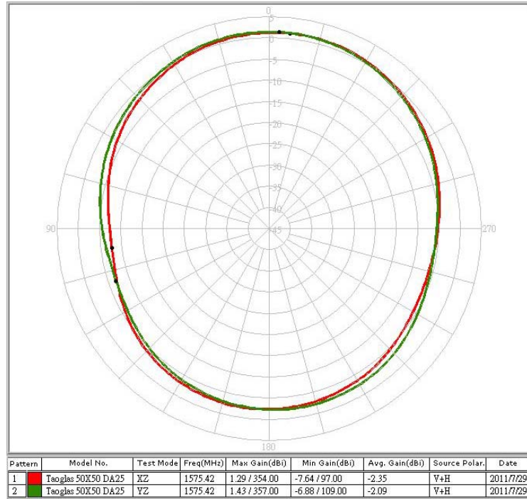
1575.4 MHz XZ+YZ-Plane
