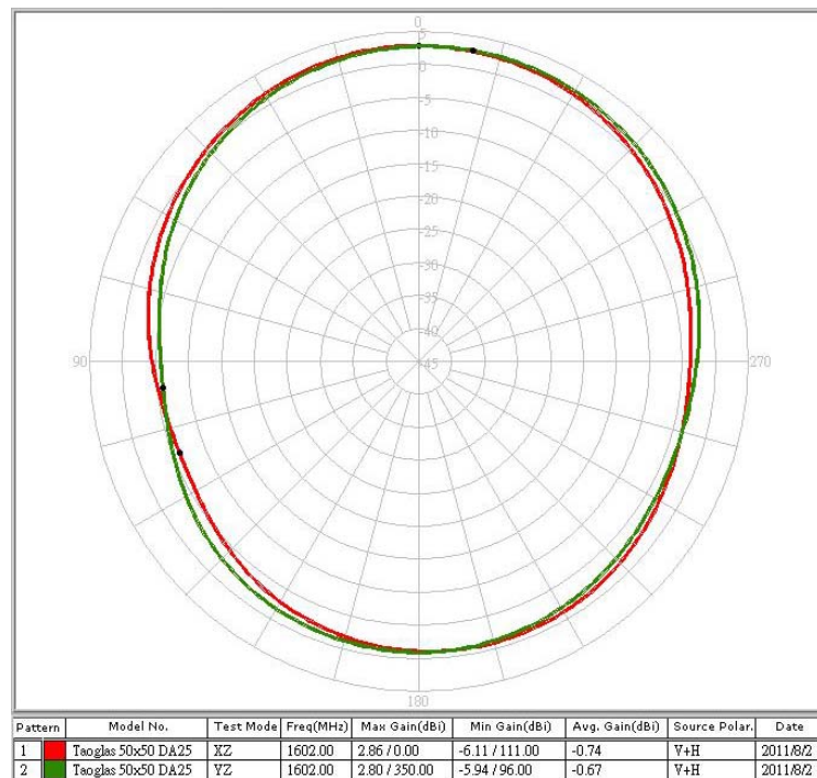
1602.0 MHz XZ+YZ-Plane
