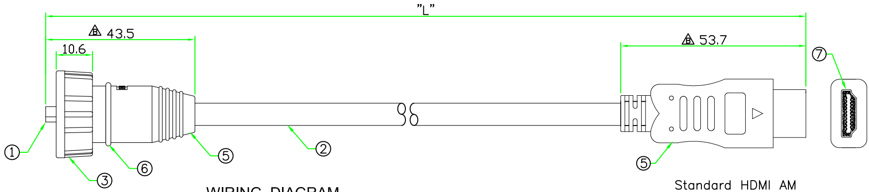
HDMI A 19P (IP66)
