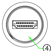
HDMI A 19P (IP66)
