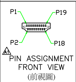
HDMI A 19P (IP66)
