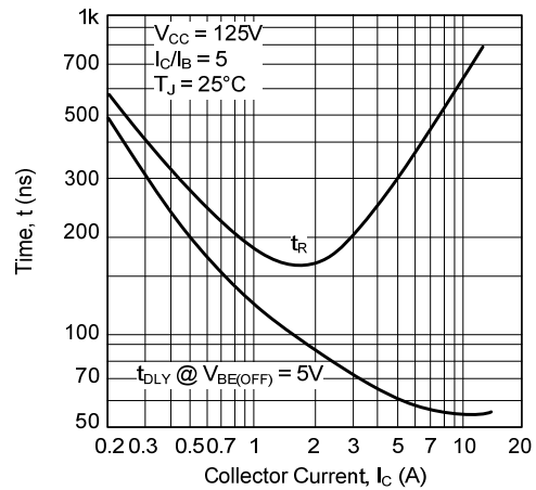
Fig. 11 Turn-On Time
