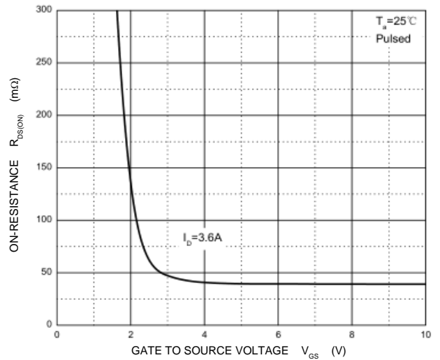
R_{DS(ON)} — V_{GS}
